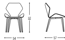
Stuhl mit Holzgestell, nicht stapelbar Chair with wooden frame, non-stackable
